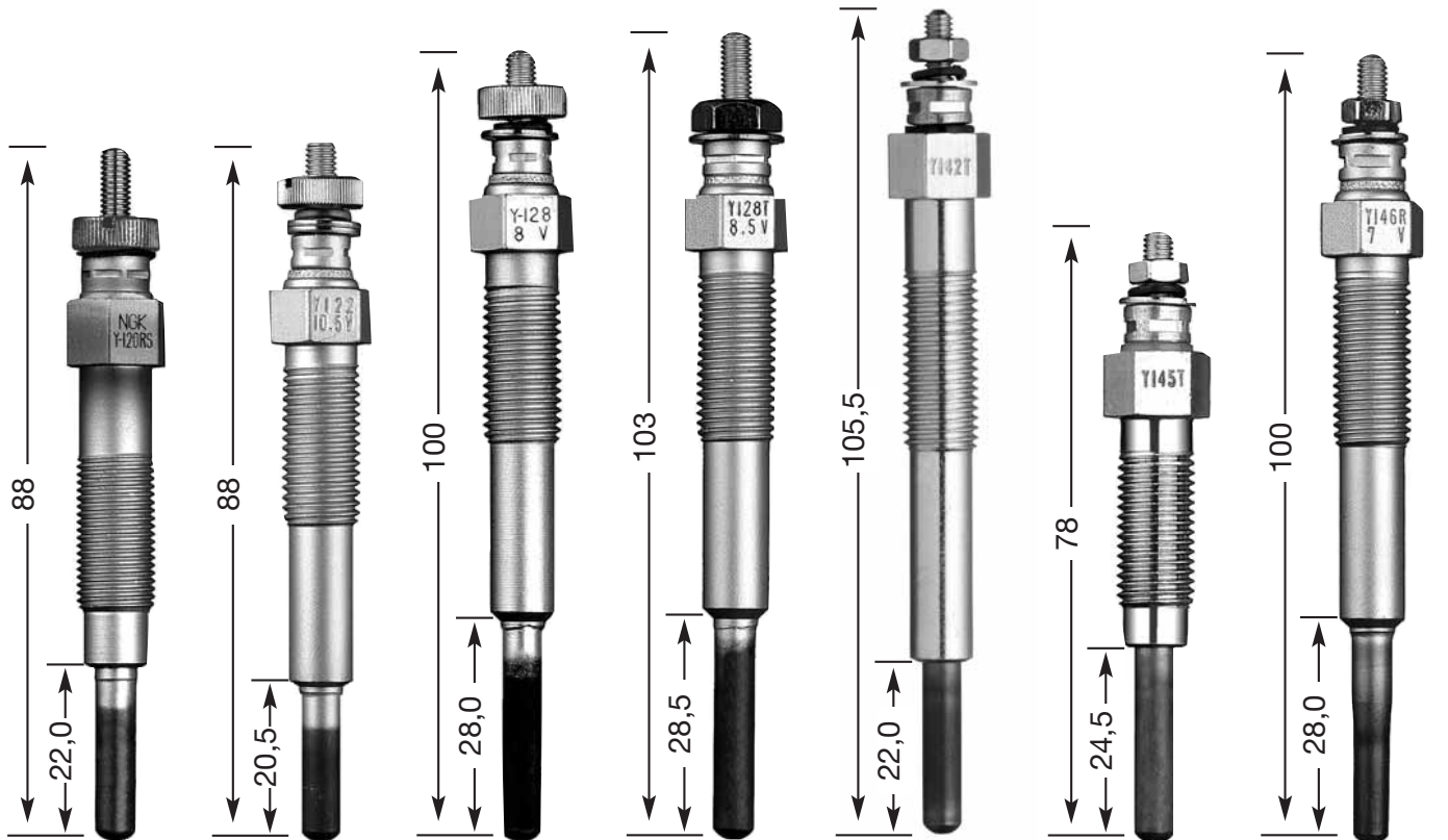
Y-120 RS M 10 x 1 12 Hex 6,5 V
