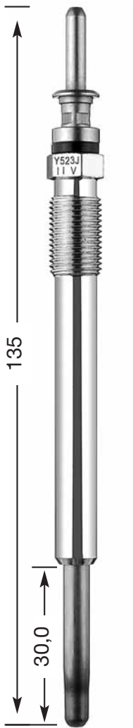
Y-523 J M 10 x 1,25 10 Hex 11 V
