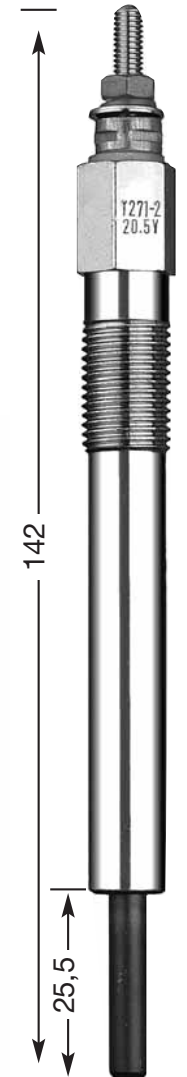
Y-271-2 M 12 x 1.25 12 Hex 20,5 V
