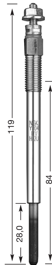
YE 04 M 8 x 1 8 Hex 11 V
