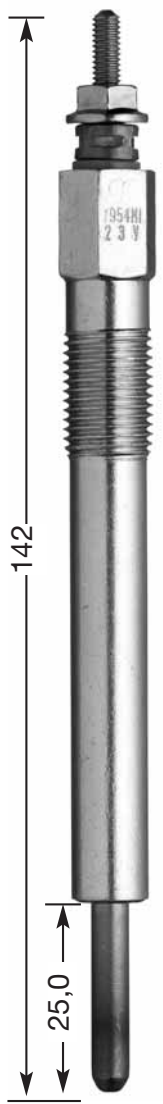
Y-954 M1 M 12 x 1.25 12 Hex 23 V
