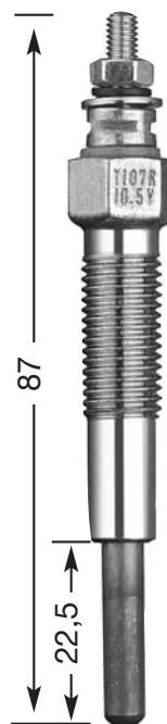
Y-107 R M 10 x 1.25 12 Hex 10,5 V
