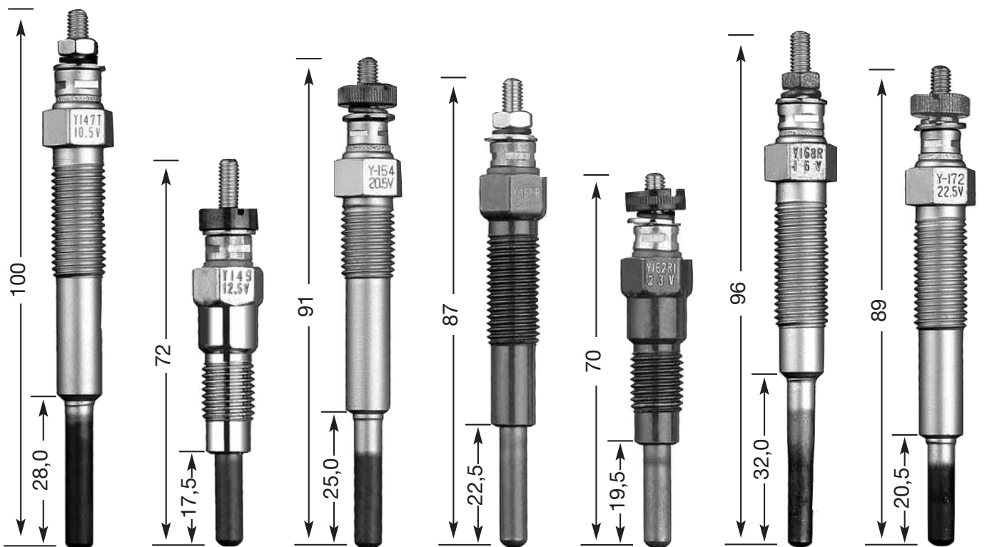
Y-147 T M 10 x 1.25 12 Hex 10,5 V
