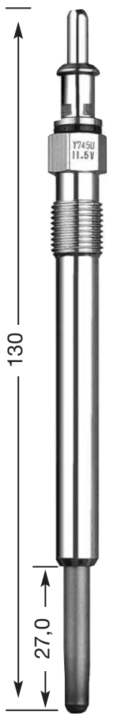
Y-745 U M 10 x 1 10 Hex 11,5 V
