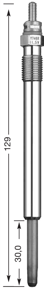
Y-746 R M 10 x 1 10 Hex 11,5 V
