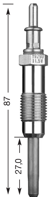
Y-929 U M 12 x 1.25 12 Hex 11,5 V
