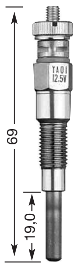
YA 01 M 8 x 1 10 Hex 12,5 V
