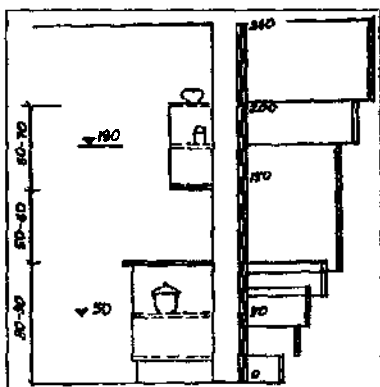
Рис. 91. Диаграмма высот рабочих поверхностей кухонного оборудования
