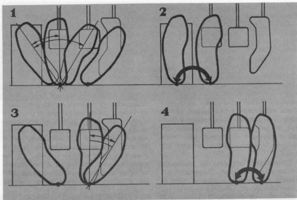
Рис. 6. Положение ног: 1 — правильное; 2 — неправильное (левая); 3 — правильное; 4 — неправильное (правая).
