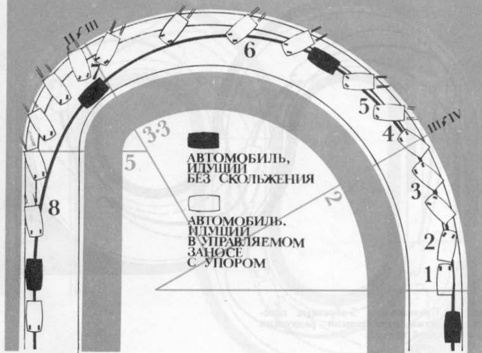
Рис. 45. Пример прохождения сложного поворота раллистами в зимних условиях: 1—подход на максимальной скорости; 2—контрсмещение (без предварительного торможения); 3—движение с малым углом заноса; 4—ударное включение третьей передачи; 5—увеличение угла заноса; 6—движение с большим углом заноса, что приводит к резкому падению скорости; 7—движение в критическом заносе; 8—выход из поворота на подъем и выравнивание автомобиля.
