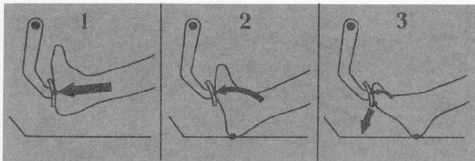
Рис. 15. Положение правой ноги на педали при торможении: 1—действие пяткой не позволяет точно дозировать тормозное усилие; 2—действие верхней частью стопы обеспечивает достаточную гамму усилий и точную их дозировку; 3—действие пальцами, хотя и точное, но не стабильное.
