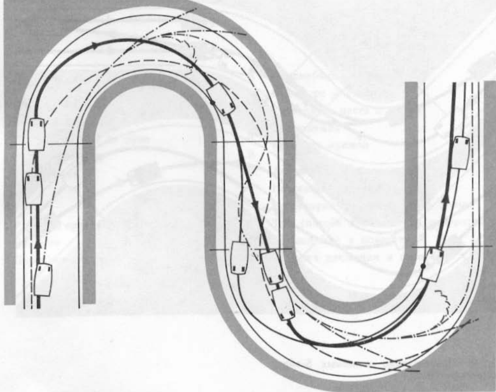
Рис. 47. Прохождение S-образных поворотов с двумя одинаковыми радиусами и переходной прямой между ними.
