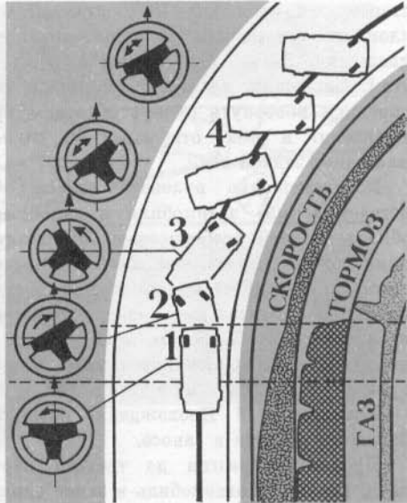
Рис. 29. Вход в управляемый занос контр-смещением: 1—вход в поворот; 2—захлестывающий дестабилизирующий маневр; 3—срыв задней оси; 4—движение в заносе.
