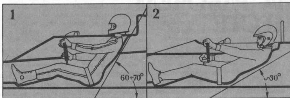
Рис. 2. Посадка спортсмена в гоночном автомобиле: 1— характерная для современных автомобилей; 2— характерная для гоночных автомобилей 60-х годов.
