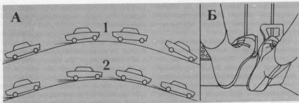
Рис. 18. Удержание автомобиля на профиле дороги. А — схема движения автомобиля: 1— без торможения; 2— с торможением (траектория повторяет профиль дороги). Б — торможение левой ногой.
