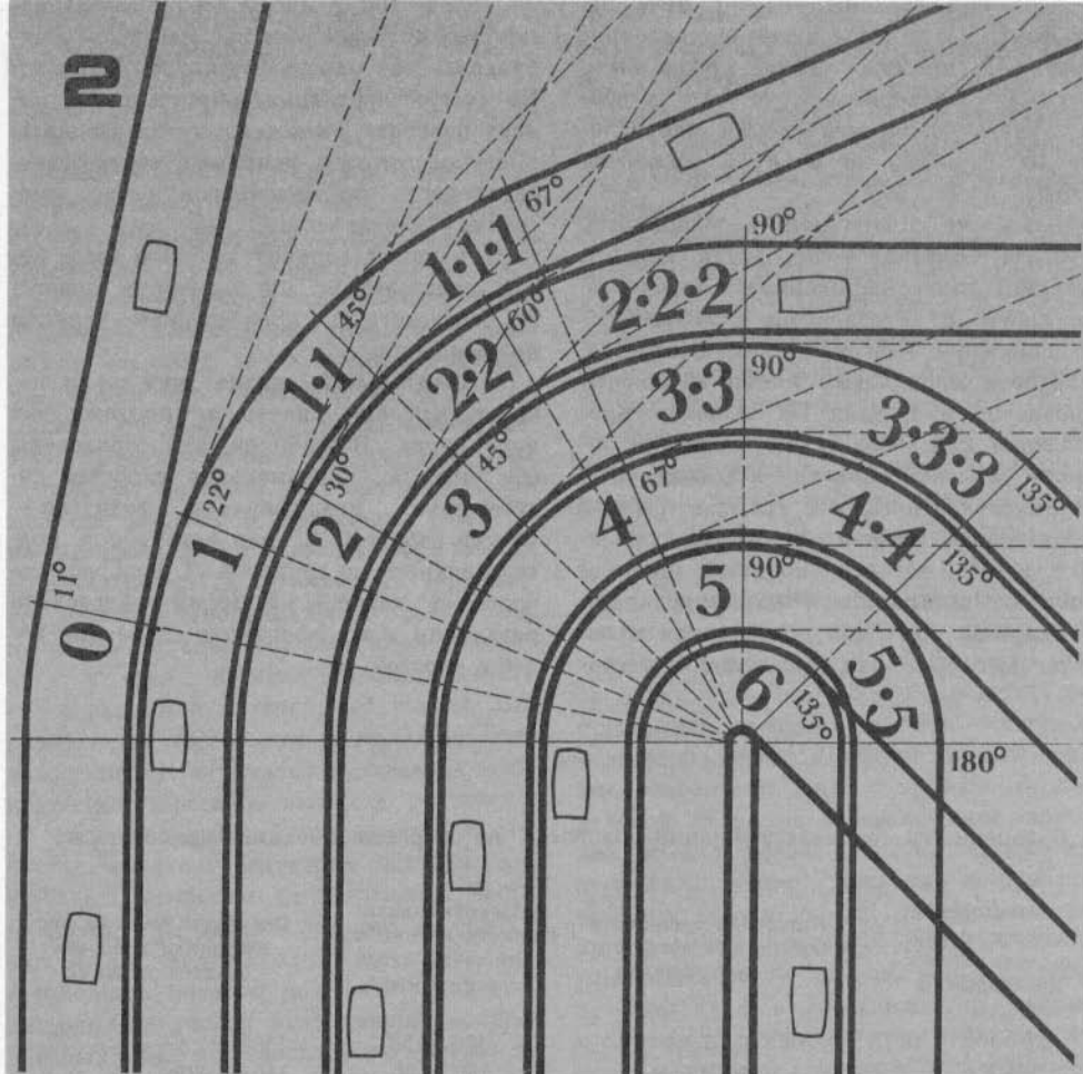
Рис. 23. Классификация поворотов: 1 — по углу; 2 — по углу и кривизне.
