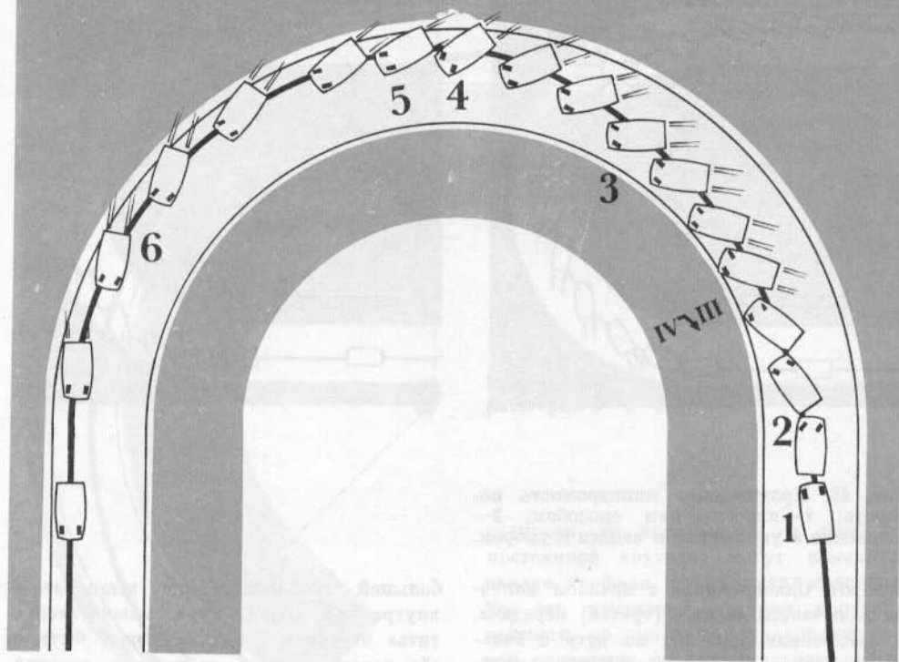
Рис. 44. Прохождение ипподромного поворота в заносе с контактным торможением: 1—подход (прямая передача, скорость — 140 км/ч); 2—контрсмещение и третья передача (без торможения); 3—движение в заносе с увеличивающимся углом; 4—касание снежного отвала задним правым крылом (колеса выворачиваются влево, «газ» не сбрасывается); 5—автомобиль разворачивает, скорость снижается, но благодаря заблаговременно вывернутым влево колесам, машина опять становится в занос, и руль возвращается в прежнее положение; 6—движение в заносе с упором колес в снежный отвал и выход.
