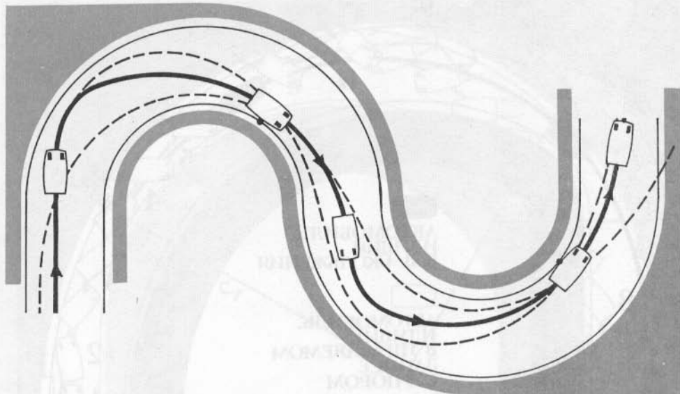
Рис. 46. Прохождение S-образных поворотов с двумя одинаковыми радиусами без переходной прямой.
