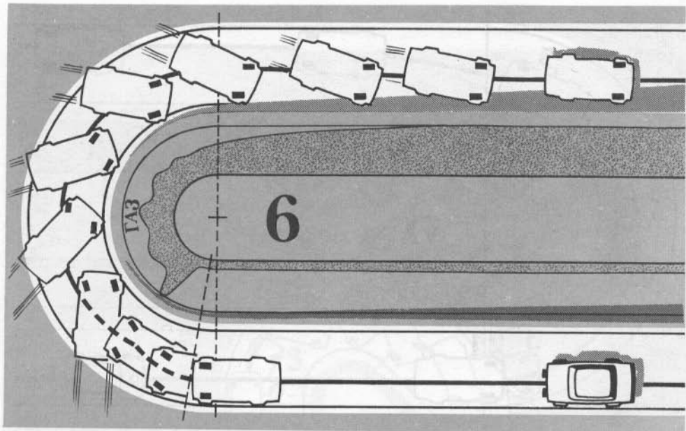
Рис. 40. Прохождение «обратных» поворотов категории 6 на спуске.
