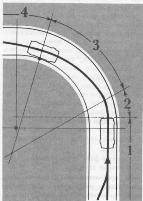
Рис. 25. Фазы прохождения поворота: 1—подход; 2—вход; 3—движение по дуге; 4—выход.
