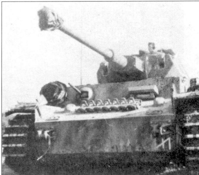
Весной 1943 года была введена новая схема камуфляжа - в качестве базового цвета в ней использовался темно-желтый. На сфотографированном среднем танке Pz.Kpfw IV Ausf F2 видны пятна старой темно-серой краски, которые особенно хорошо заметны на переднем броневом листе корпуса. Обратите внимание, что дивизионная эмблема - «волчий капкан» (wolfsangel) для лучшей заметности нарисована белой краской.
