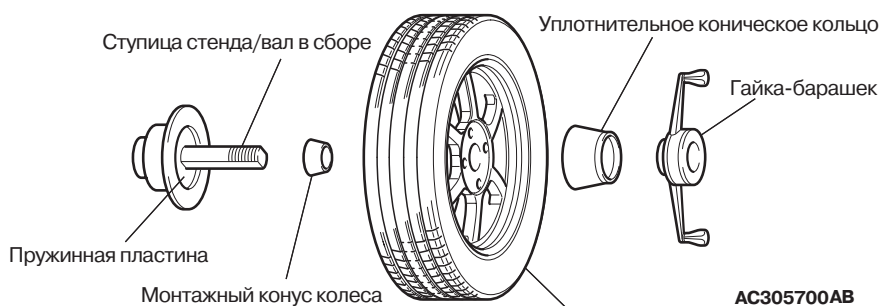
Колесо в сборе стандартного легкового автомобиля
