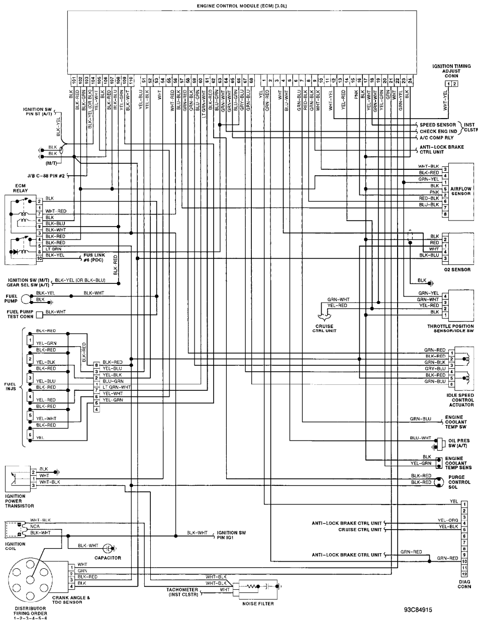
Fig. 1: Wiring Diagram (3.0L)
