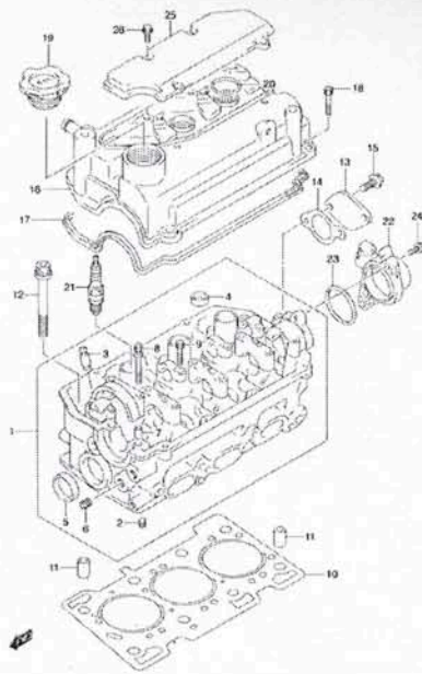
DASZT.2.003 CYLINDER HEAD (4V)
