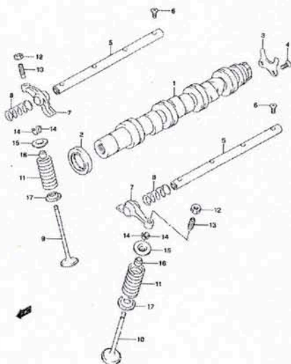
Camshaft-Valves (Turbo)
