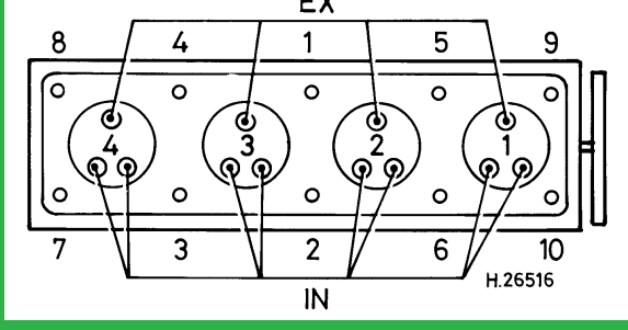
1995 cm³, 12V
