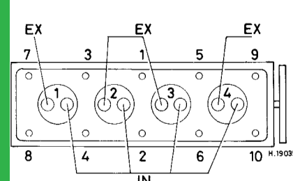
2316 cm 3 , 8V
