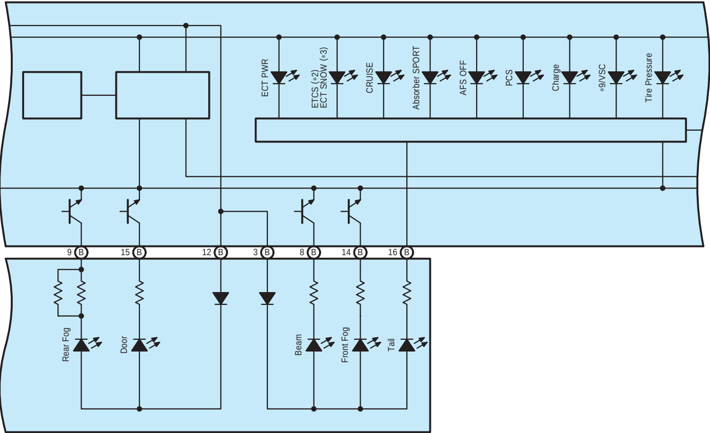
z2(B) Telltale Lamp Assembly
