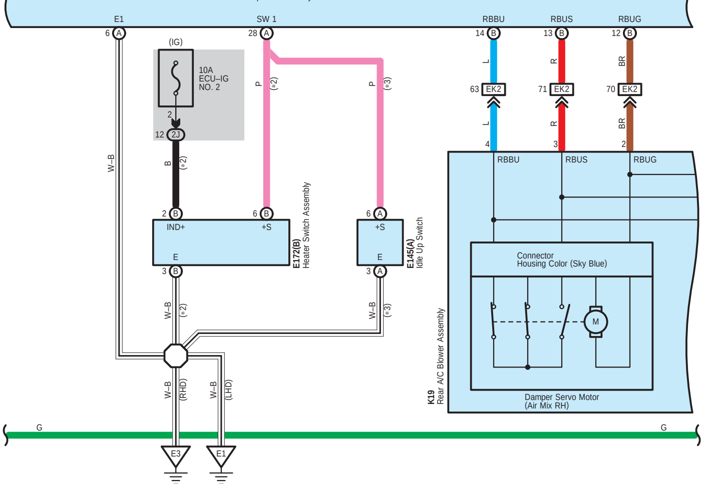
E35(A), E36(B), z66(C) A/C Amplifier Assembly
