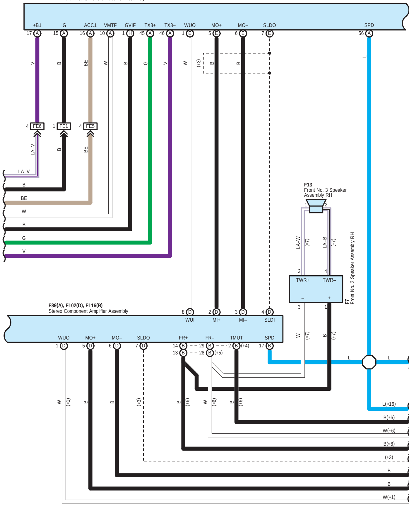
F76(A), F77(B), F96(C), F101(E), F103(D), F104(I), F105(H), F108(F), F117(G) Multi-Media Module Receiver Assembly
