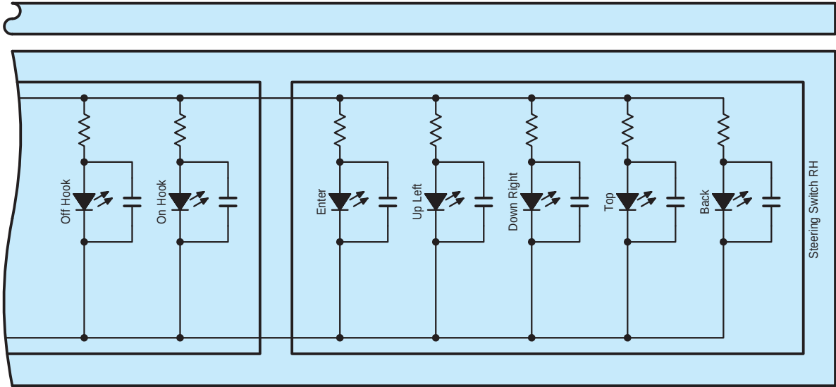
z65(D) Steering Pad Switch Assembly
