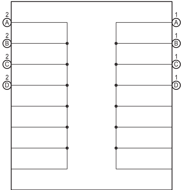
O152(A), O153(B), O154(C), O155(D) No. 13 CAN Junction Connector
