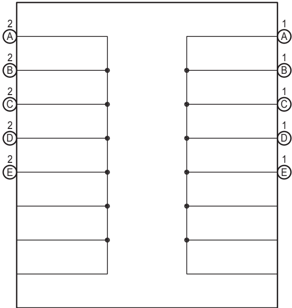
O156(A), O157(B), O158(C), O159(D), O160(E) No. 14 CAN Junction Connector
