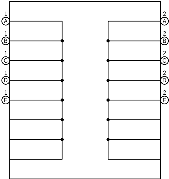
O180(A), O181(B), O182(C), O183(D),O184(E) No. 14 CAN Junction Connector
