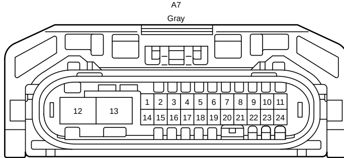
90980-12A92
