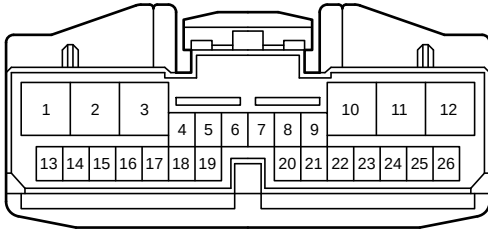
82824-12510
