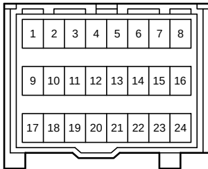
90980-12392
