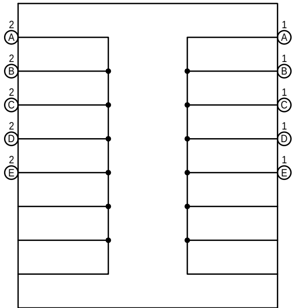
O157(A), O158(B), O159(C), O160(D), O161(E) No. 12 CAN Junction Connector
