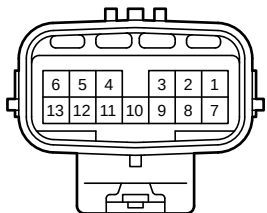
90980-12716
