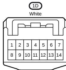
90980-12370
