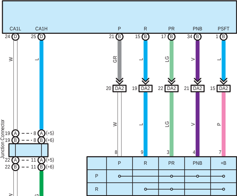
D15 Shift Lever Position Sensor
