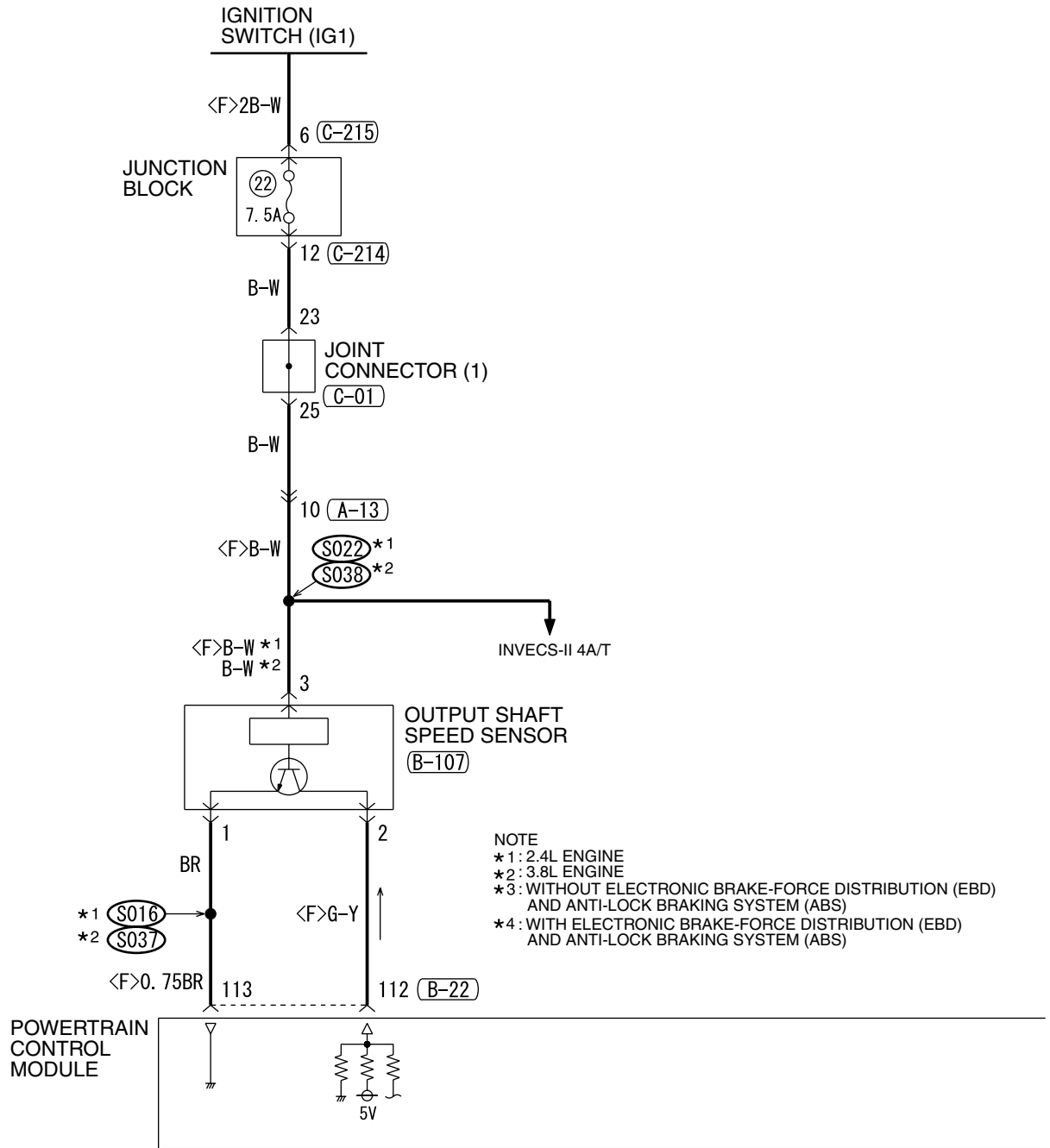
(A-13)
