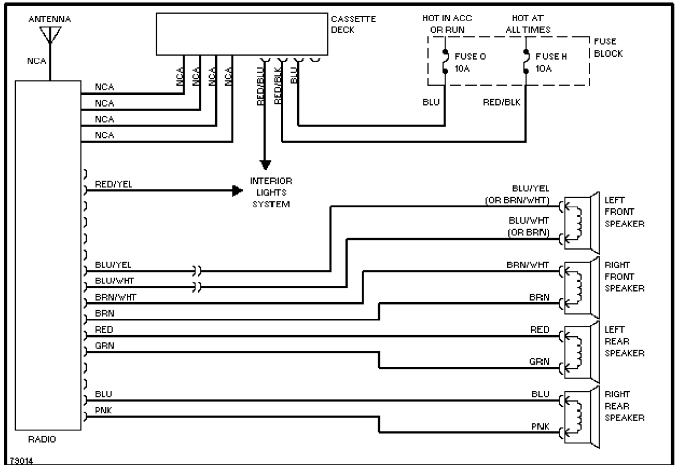
Radio Circuits
