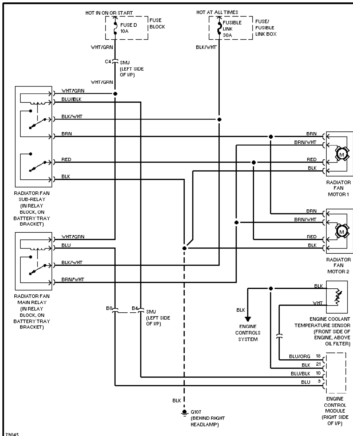
1.6L, Cooling Fan Circuit, A/T
