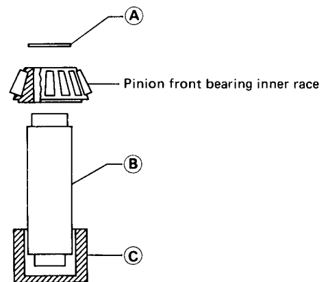
SPD534
