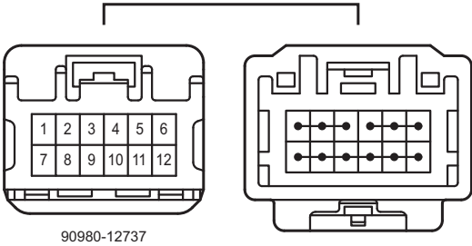
G80 Black
