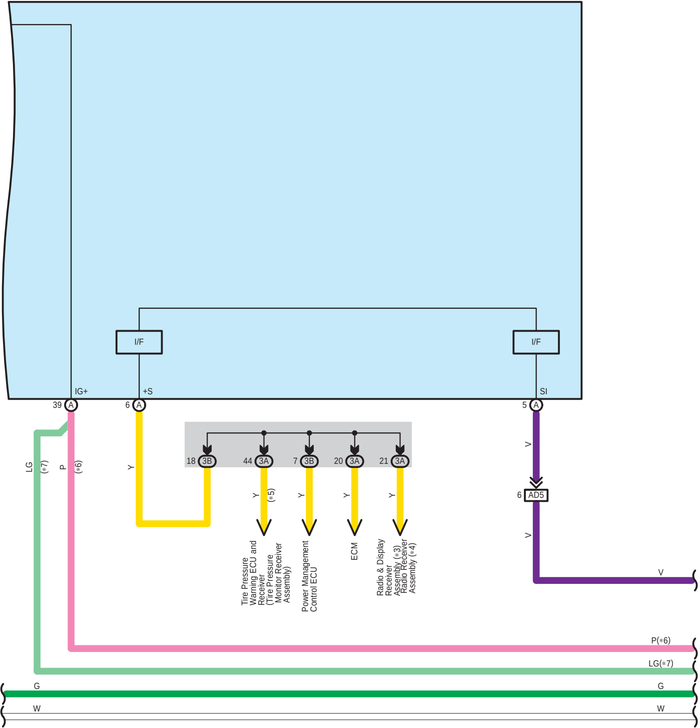
D66(A), D141(B) Combination Meter
