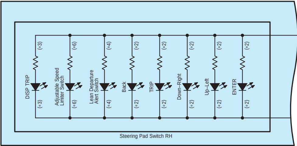
z24(D) Steering Pad Switch Assembly
