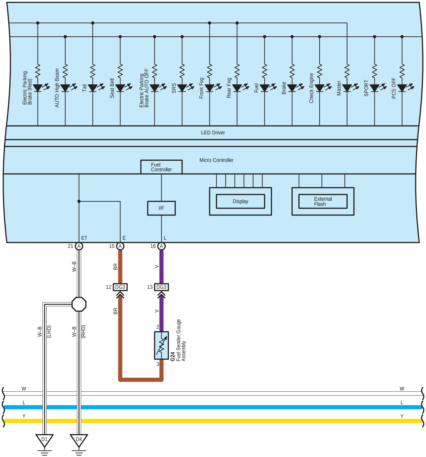
D66(A), D140(B) Combination Meter
