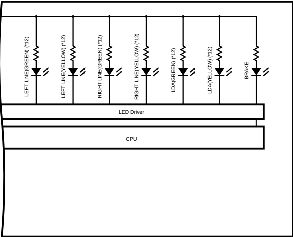
E12(A) Combination Meter Assembly
