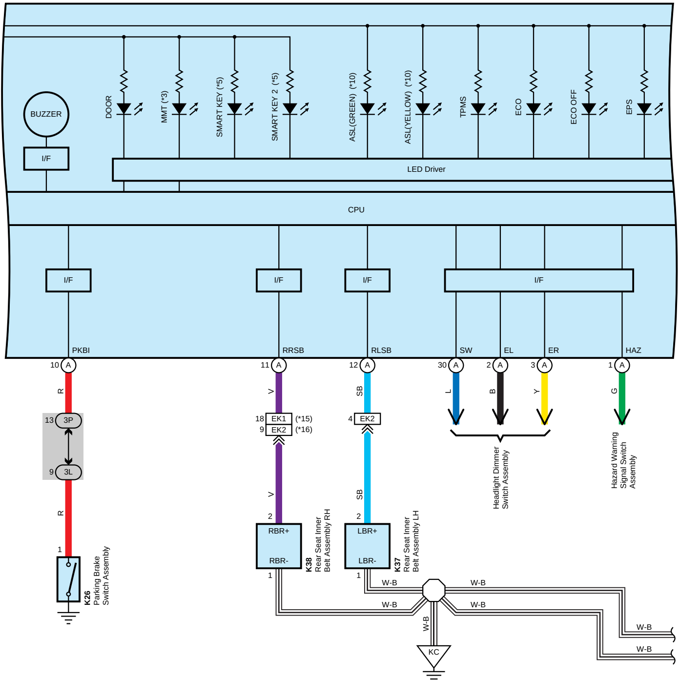
E12(A), E13(B) Combination Meter Assembly
