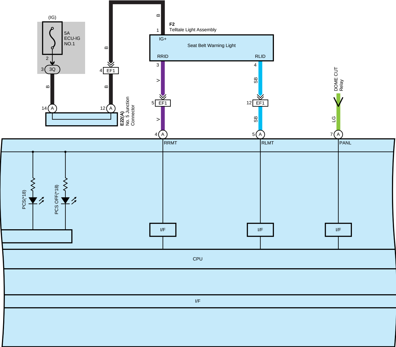
E12(A), E13(B) Combination Meter Assembly
