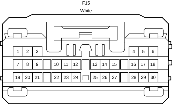
90980-12909
