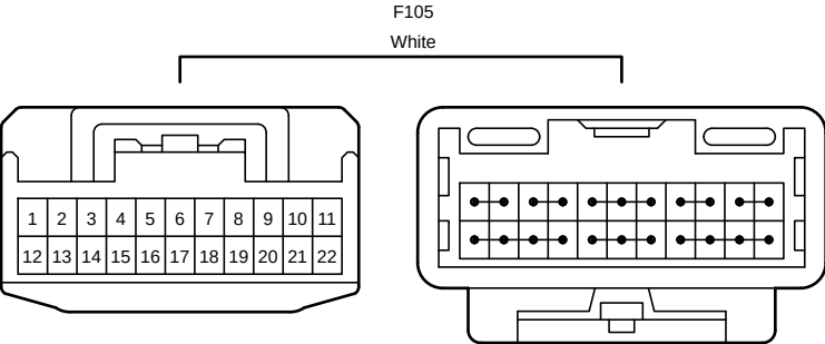
90980-12372
