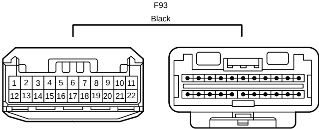
90980-12B54
