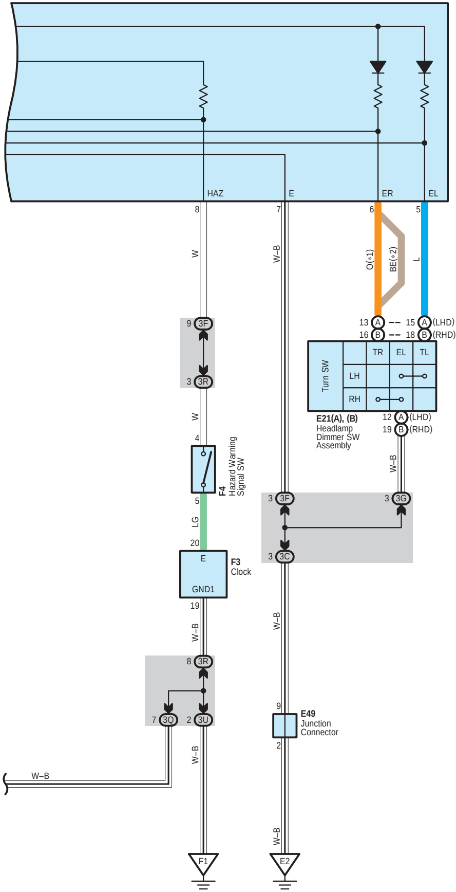
E14 Turn Signal Flasher
