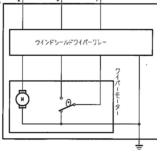
④ リヤワイパーモーター & リレー
