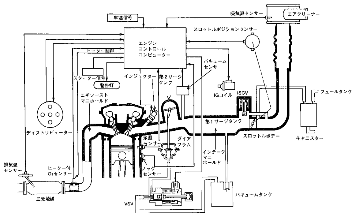
制御システムシステム
