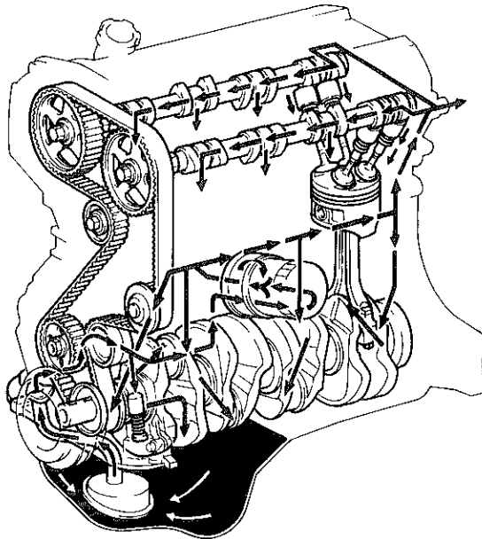
潤滑系統
