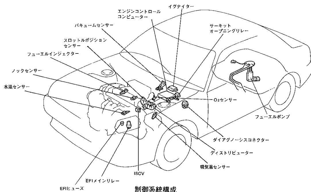
制御系統構成
