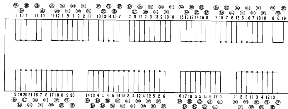
J/B No.3(内部回路)
