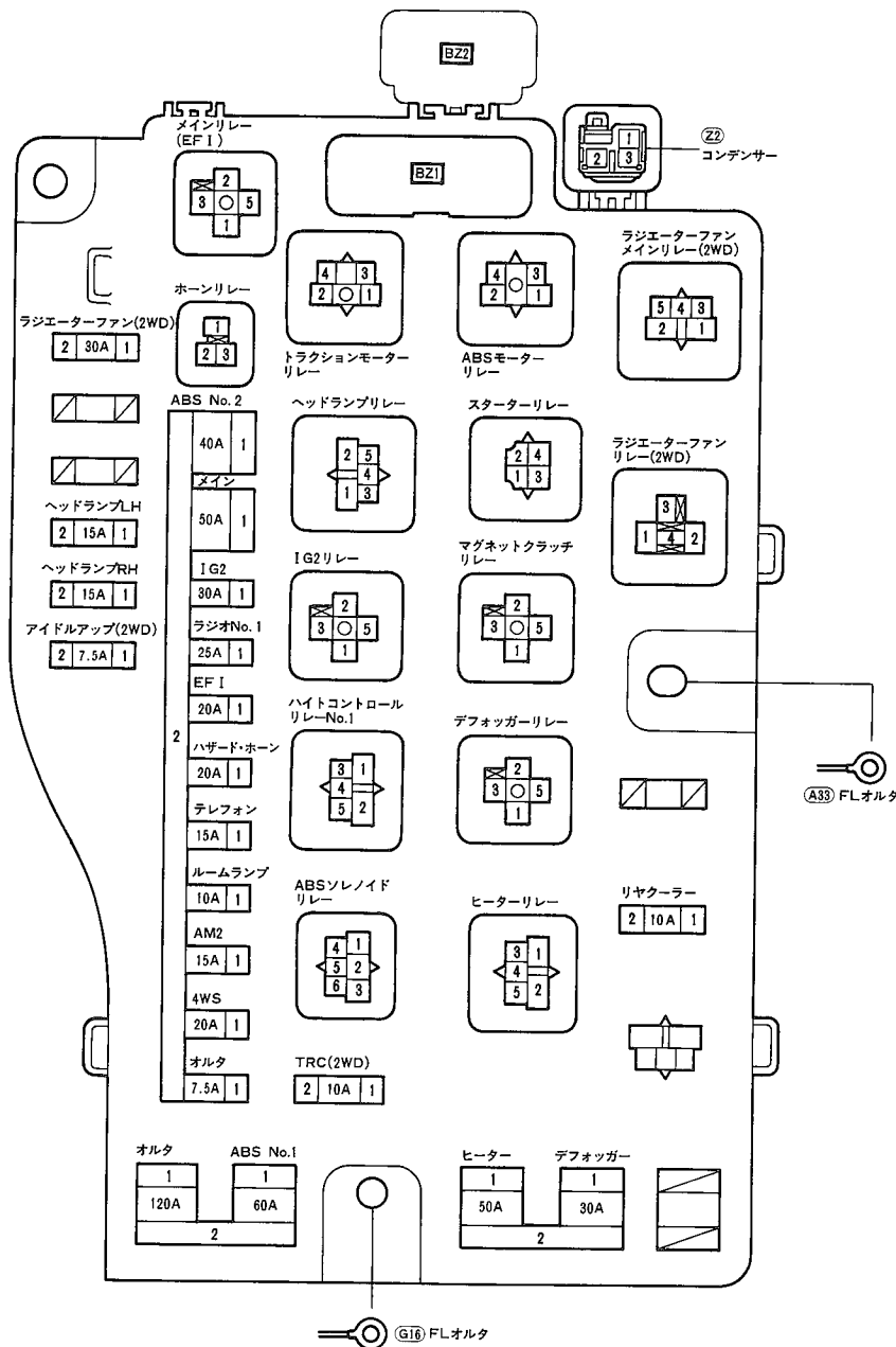
R/B No.2(エンジンルーム左)
