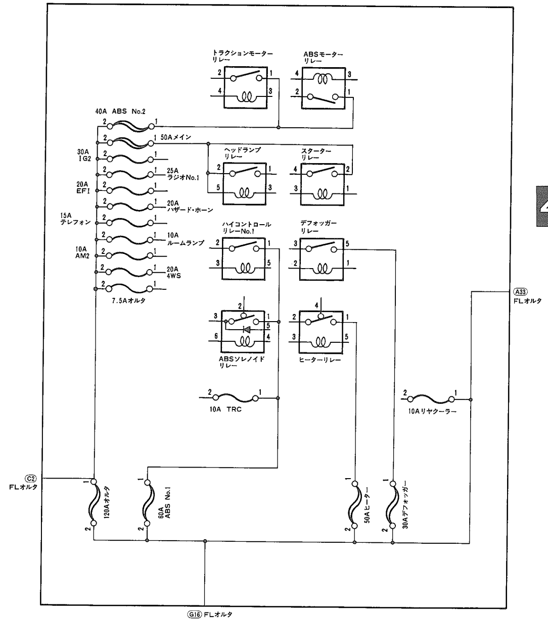
R/B No.2(内部回路)
