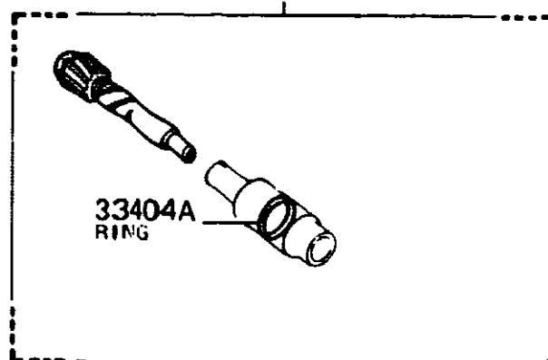
33403 GEAR
