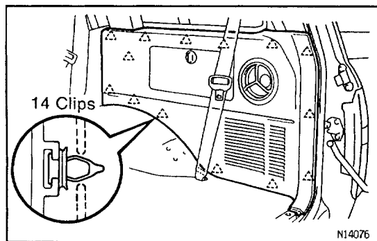
(d) Quarter trim (RH)
