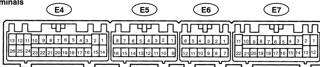
ECM Terminals
