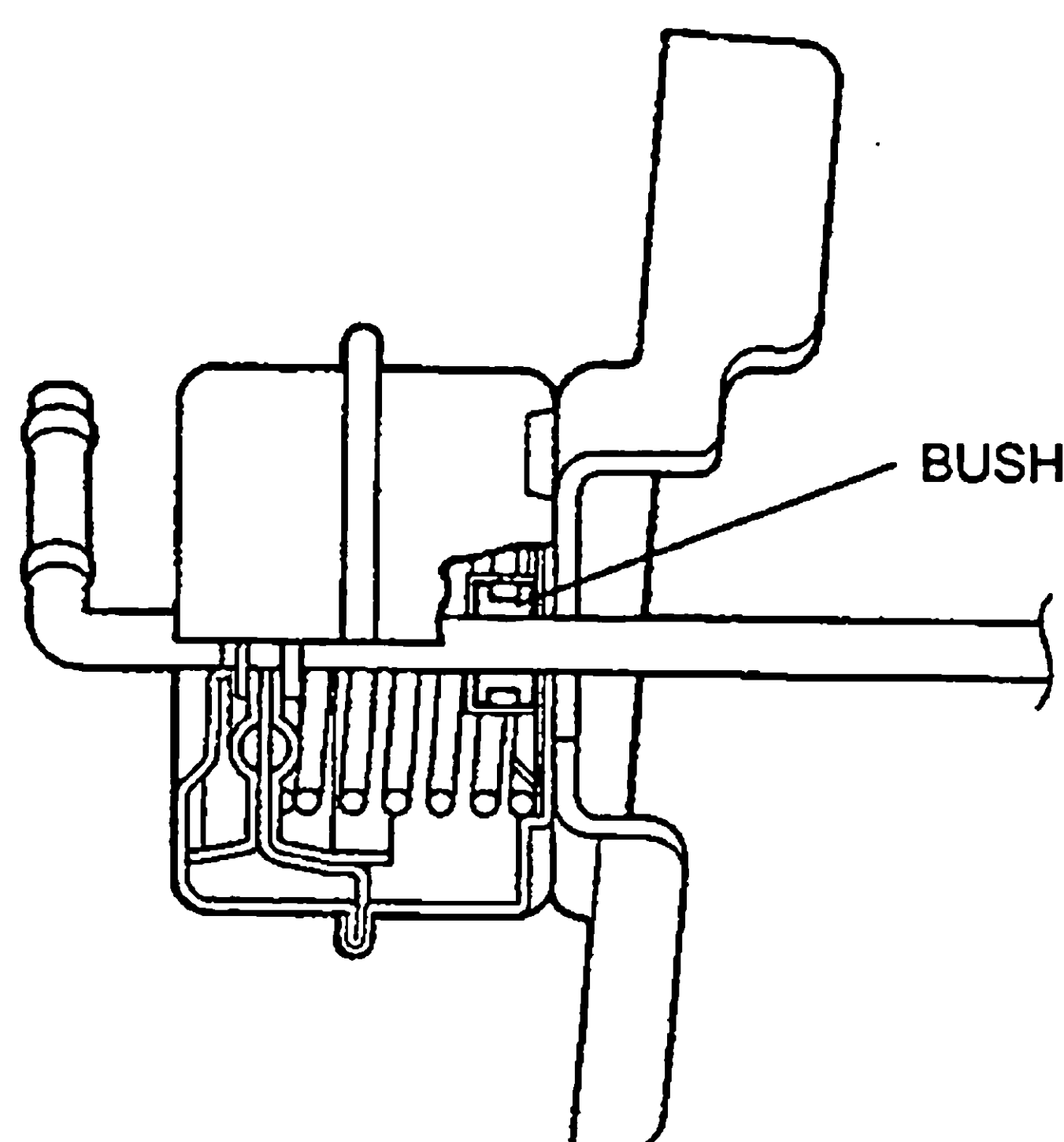
ACTUATOR
