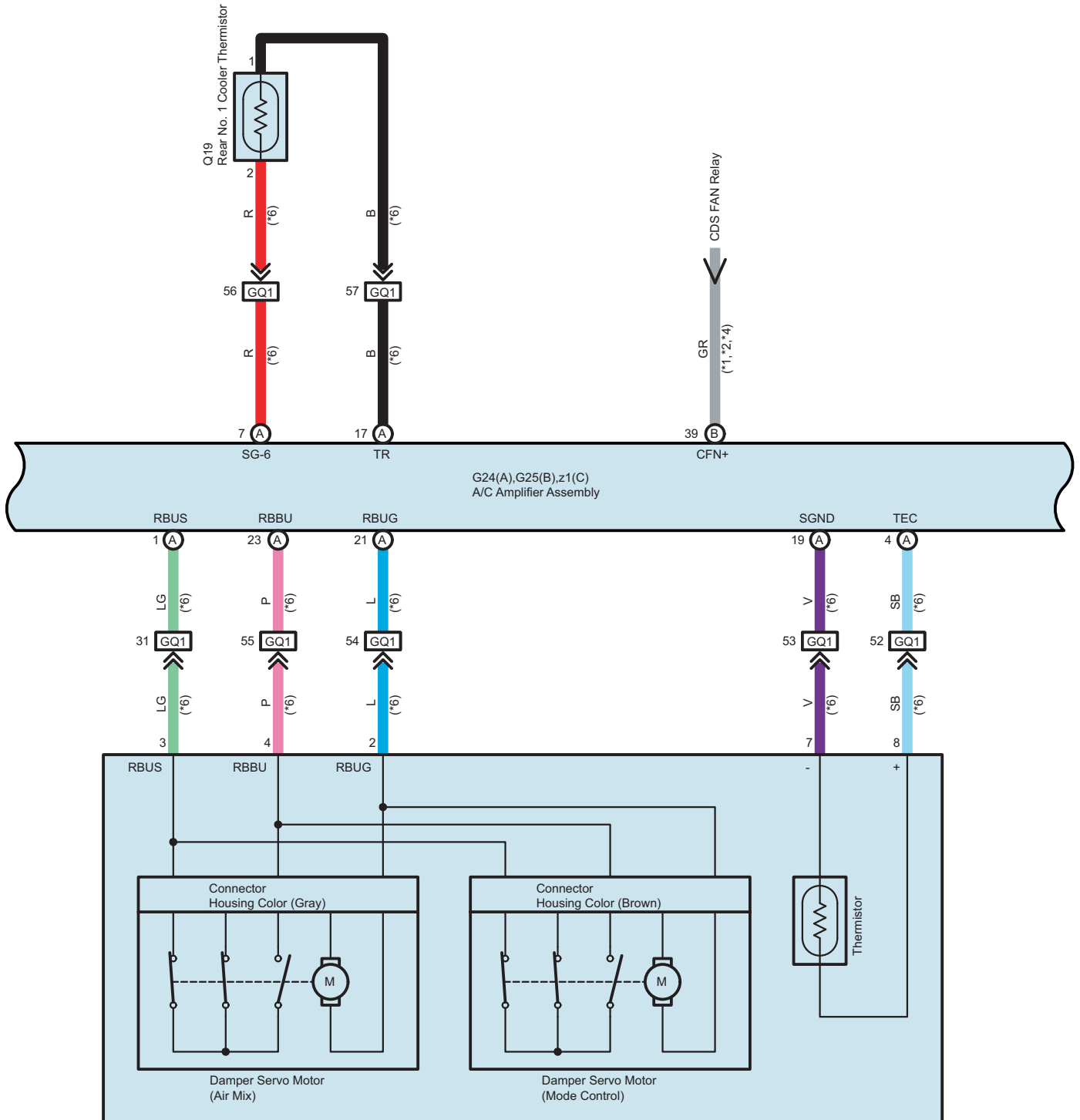
Q13 Rear A/C Blower Assembly
