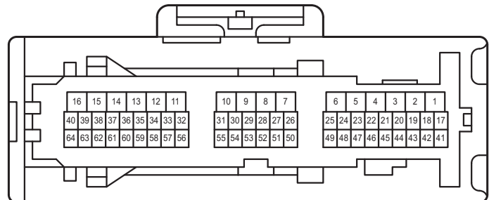
90980-12798
