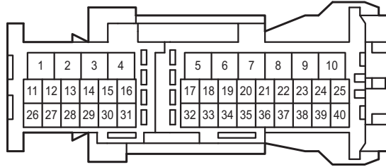
90980-12794
