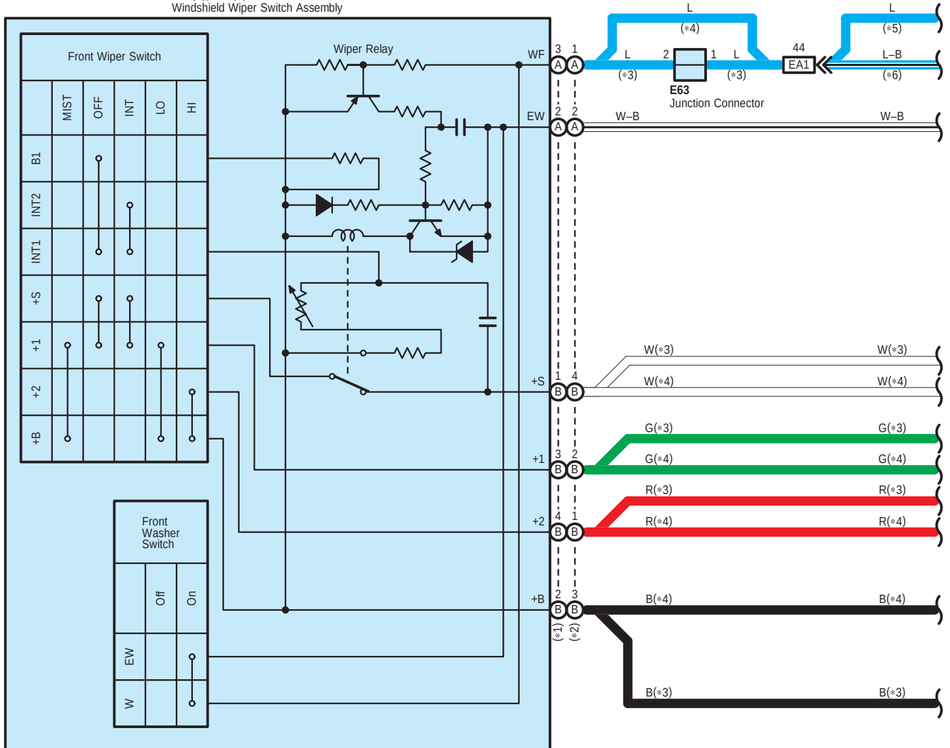
E15(A), E16(B) Windshield Wiper Switch Assembly
