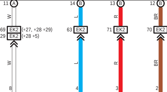
E35(A), E36(B), E81(D), E165(C), z71(E), z72(F) A/C Amplifier Assembly
