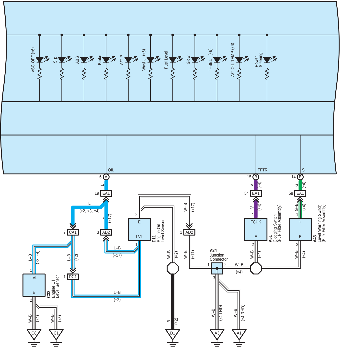
E7(A), E8(B) Combination Meter Assembly
