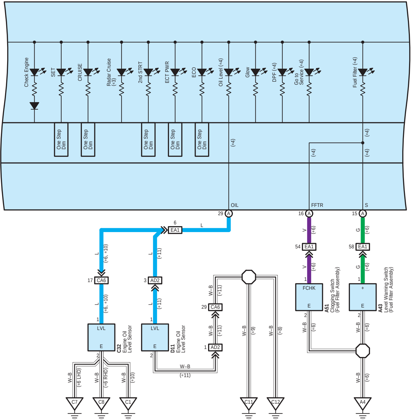
E119(A), E120(B) Combination Meter Assembly
