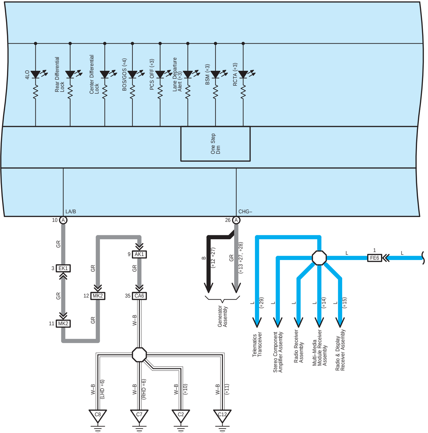
E119(A), E120(B) Combination Meter Assembly
