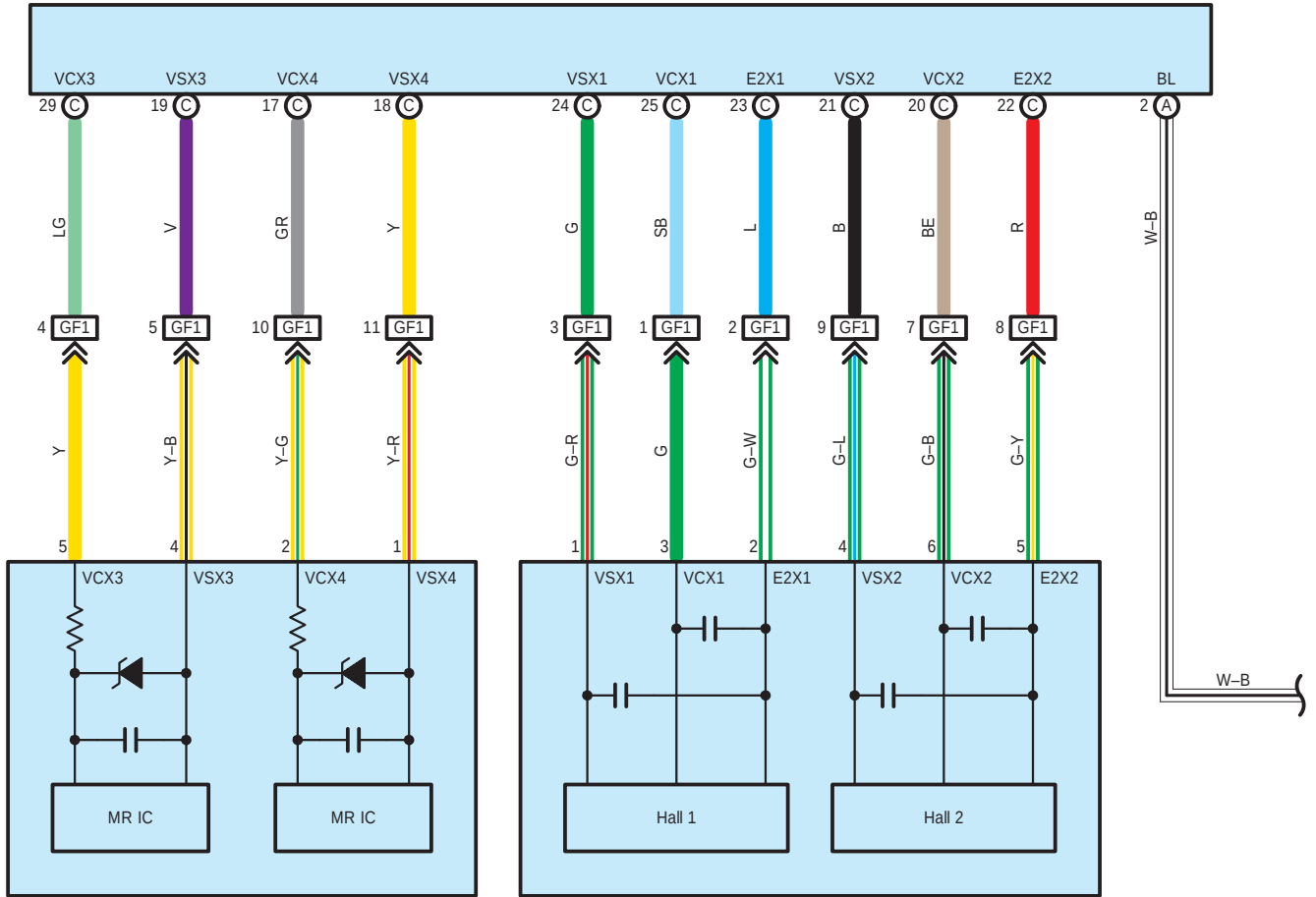
F1 No. 2 Shift Lever Position Sensor
