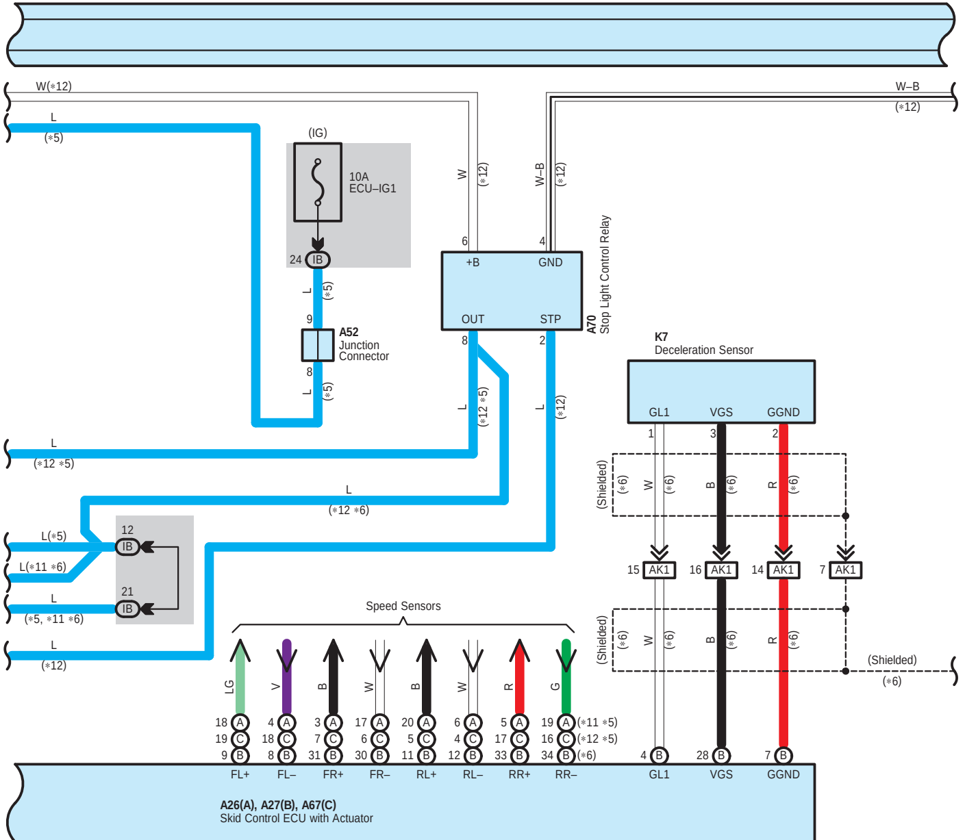
E75(A), E87(B), E111(C), E112(D) Junction Connector
