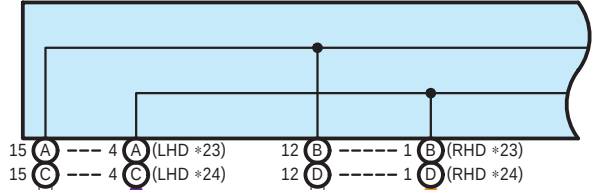
E75(A), E87(B), E111(C), E112(D) Junction Connector
