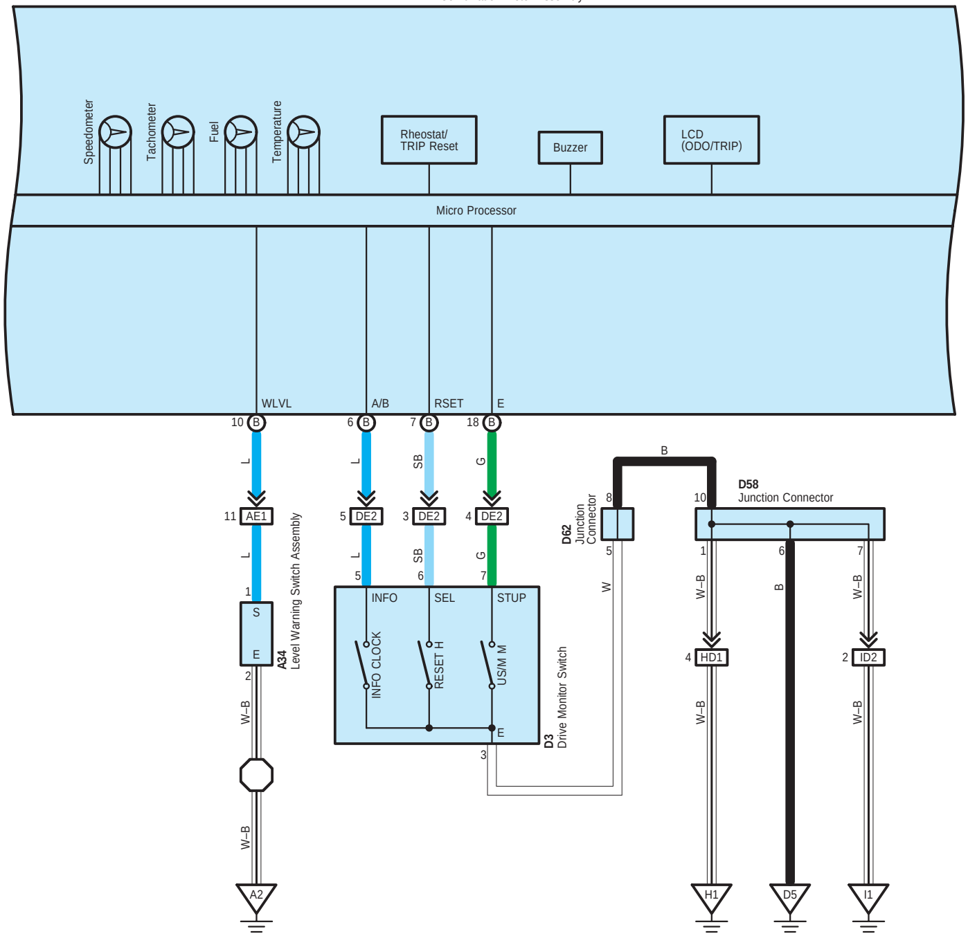
E1(A), E2(B) Combination Meter Assembly
