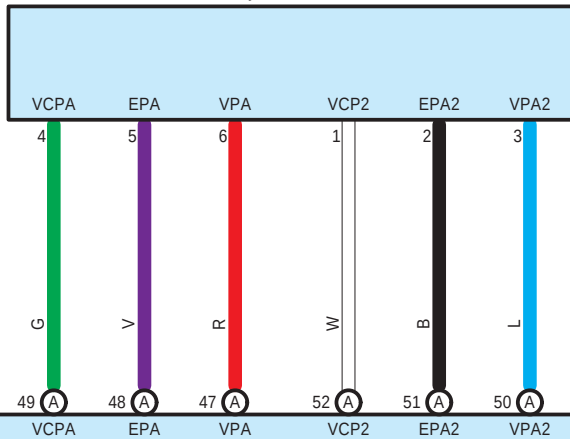
A58(A), B112(C), B118(D) ECM
